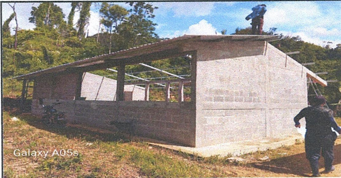
FOTOGRAFIA 1: Instalacion de la cubierta de lamina troquelada cal 26.
